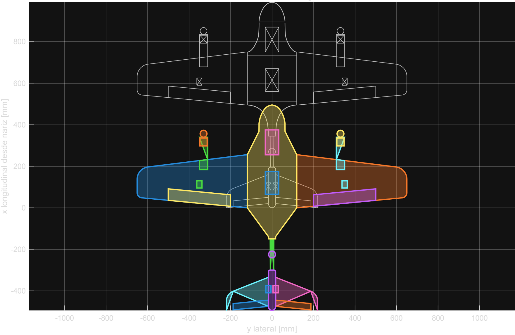
Partes DXF sobre silueta general
